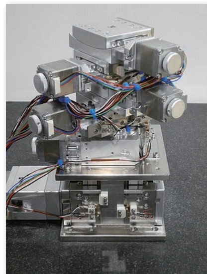
高真空対応 6 軸ステージ
